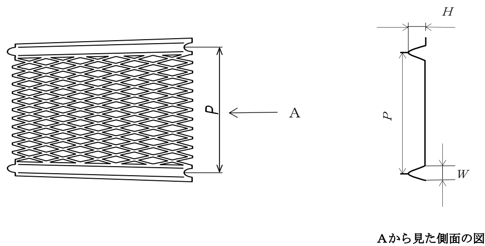
図 4ーリブラス A の例
