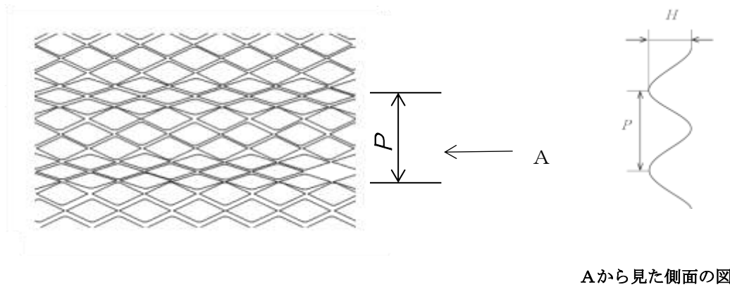
図 3－波形ラスの例
