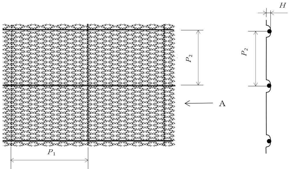
図 6－力骨付きラスの例 A から見た側面の図
