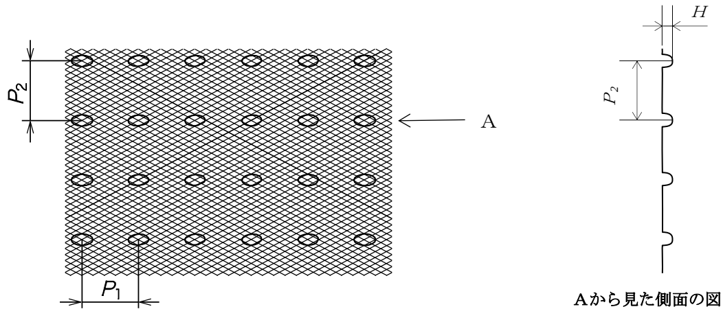
図 2—こぶラスの例
