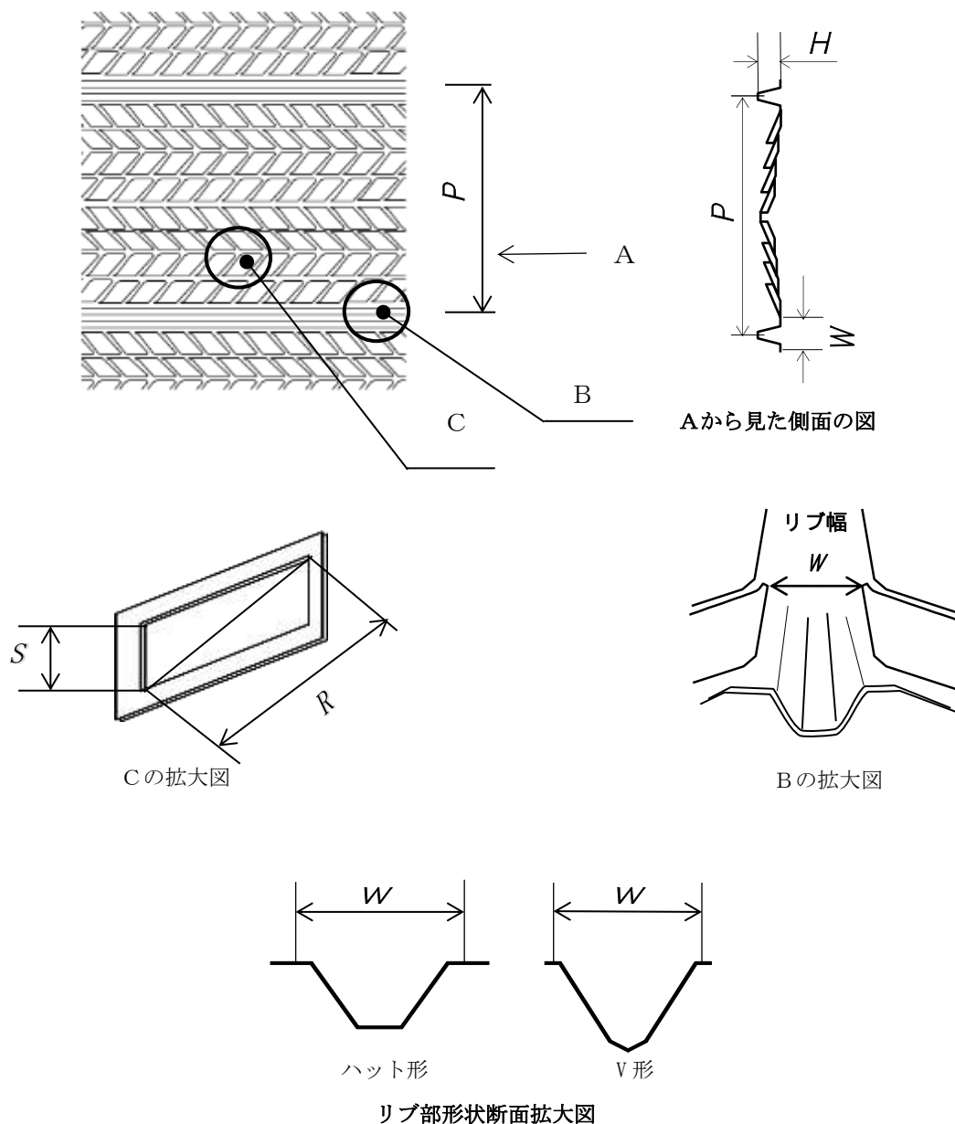
図 5-リブラス C の例
