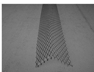
コーナー用ラス 90 × 90 × 1829mm
